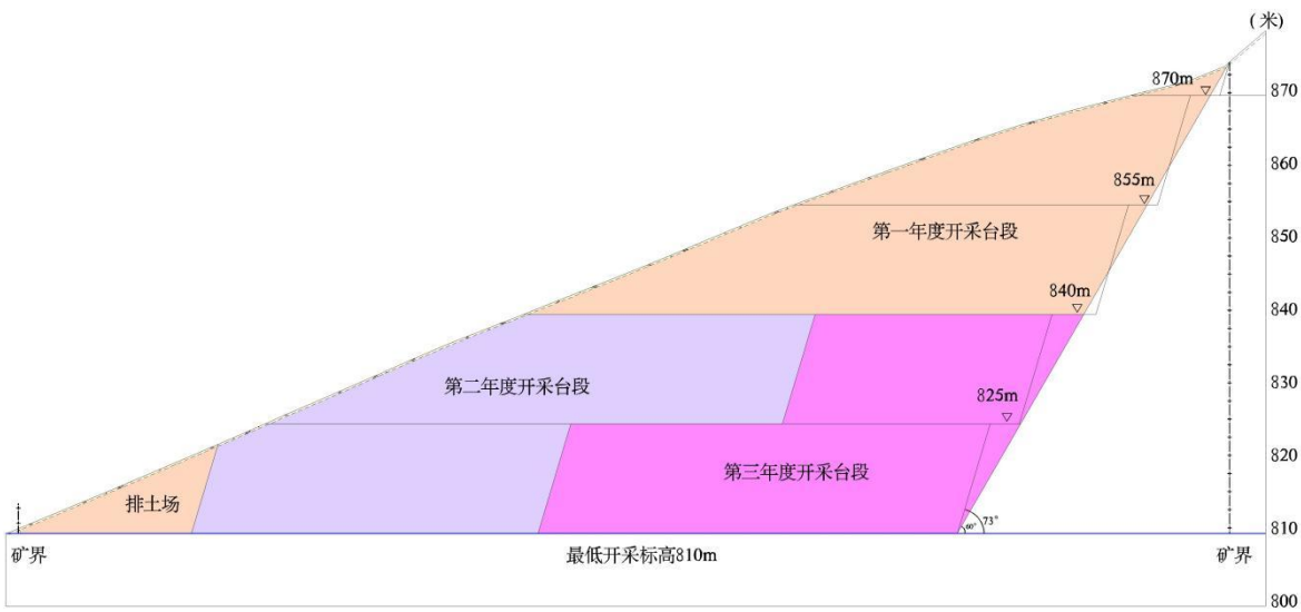
图 3-4 矿山采矿时序示意图
