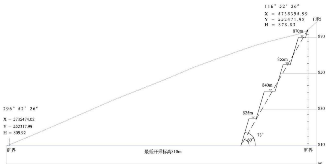
图 1-4 开采终了示意图
