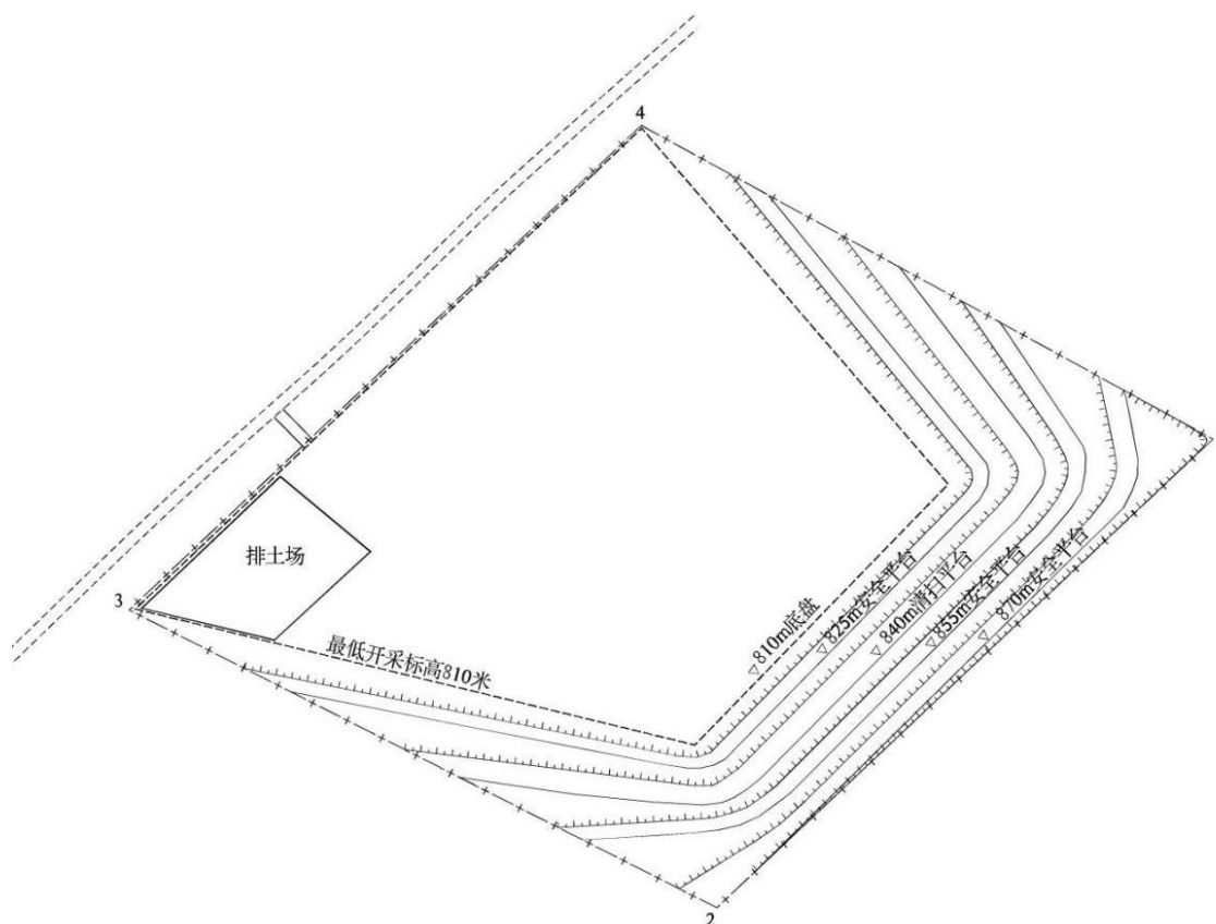
图 1-5 矿区开采平面示意图
